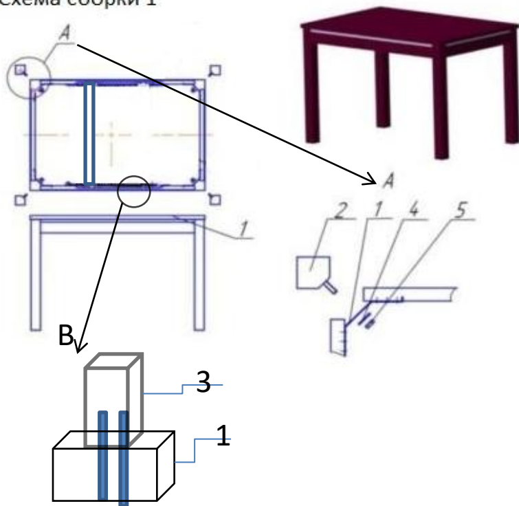
Схема сборки 1
