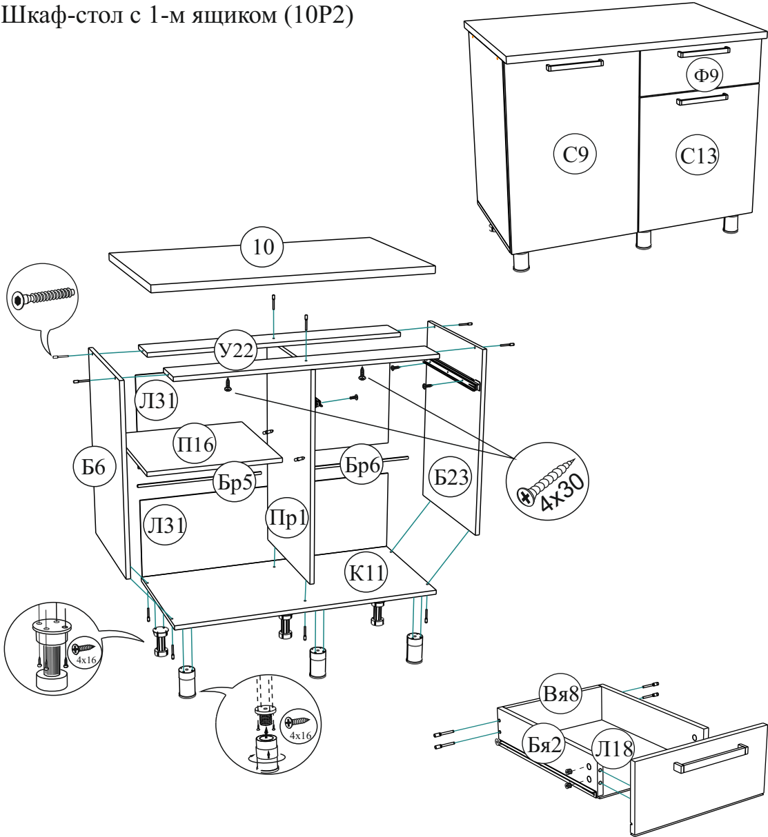
порядок сборки ящика - см. схему №1
