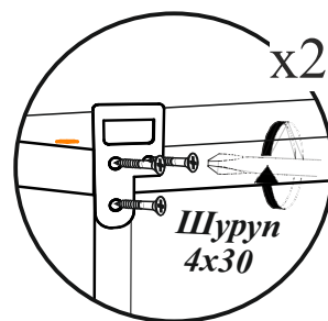
Схема навеса полки
